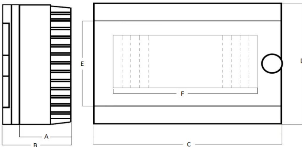
DIMENSIONS
